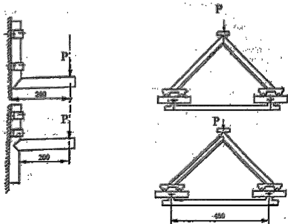
Рисунок 4 - Определение прочности угловых сварных соединений (для углового соединения под 90° и Т-образного соединения)
