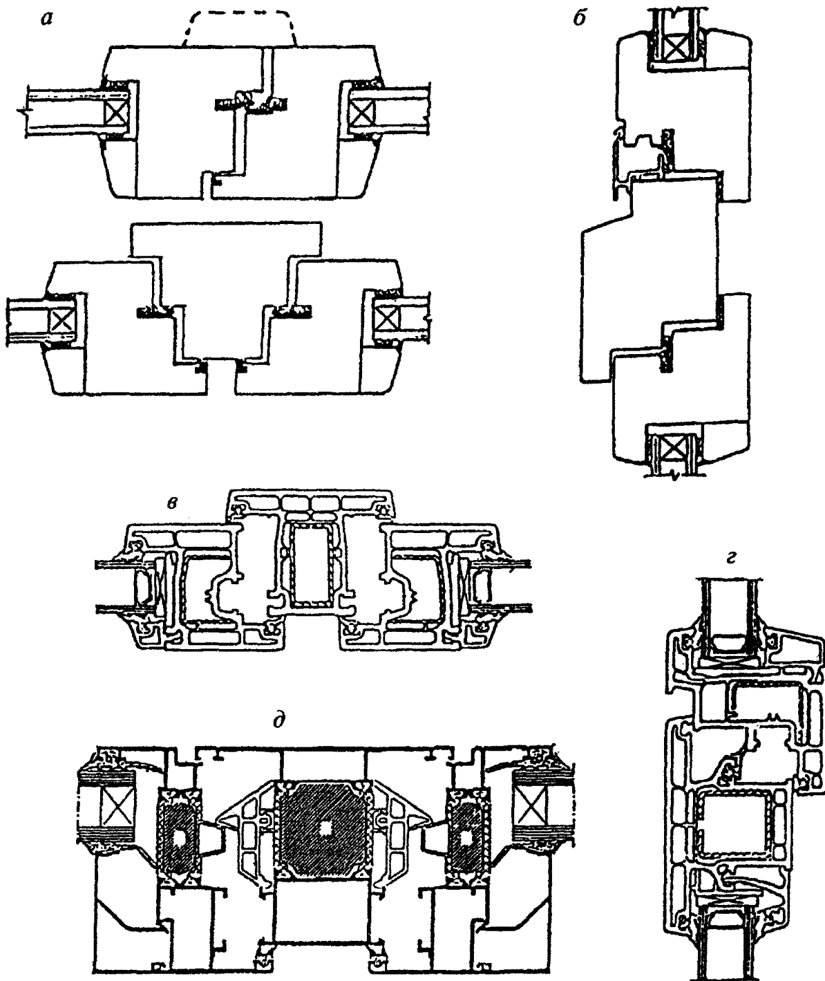
а — вертикальные безимпостный (штульповой) и импостный притворы деревянного оконного блока; б — горизонтальный импостный притвор деревянного оконного блока; в — импостный притвор оконного блока из ПВХ профилей; г — узел импостного соединения открывающейся створки и остекленной коробки; д — импостный притвор оконного блока из алюминиевого сплава
