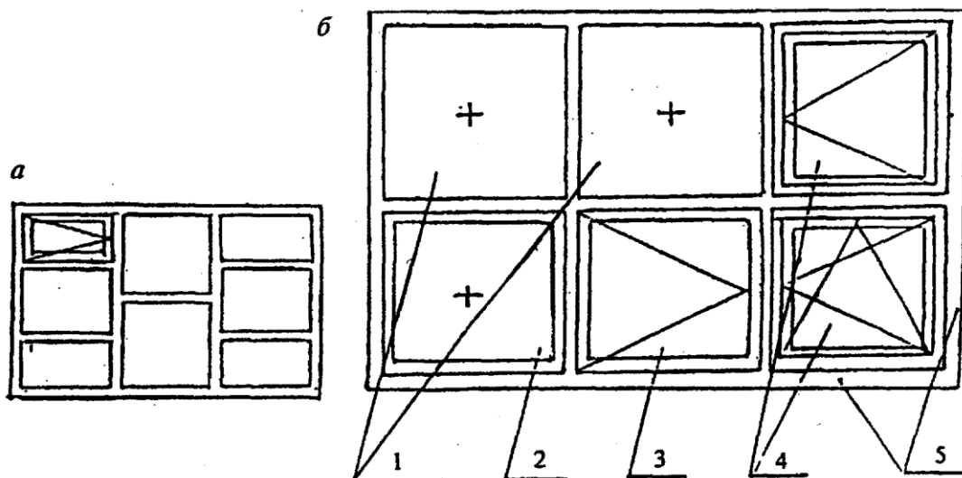
а — пример деревянной оконной рамы для остекления веранды; б — пример металлической рамы с различными видами заполнения конструкции: 1 — стеклопакетами;
