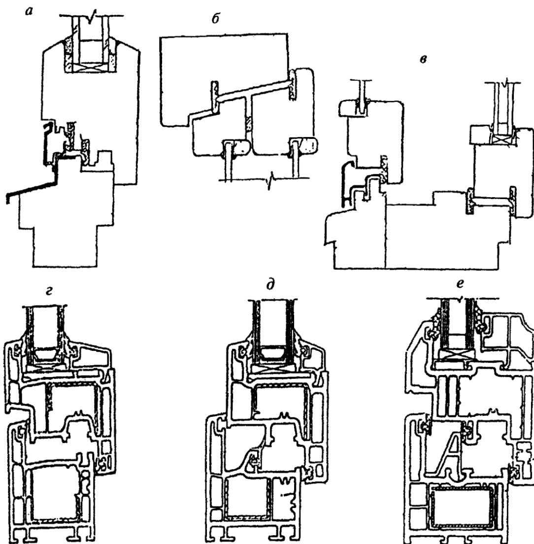
a — конструкция с двумя средними уплотнениями; б — конструкция со средним и внутренним уплотнениями; в — конструкция с двумя средними и внутренним уплотнениями; г — конструкция с наружным и внутренним уплотнениями; д — конструкция со средним и внутренним уплотнениями; е — конструкция с наружным, средним и внутренним уплотнениями
